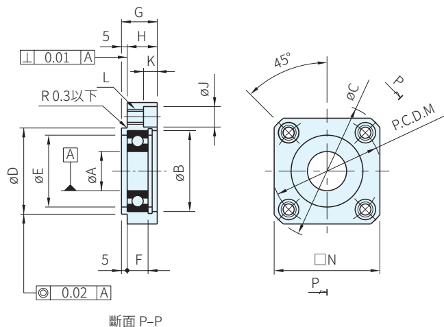
斷面 P-P
